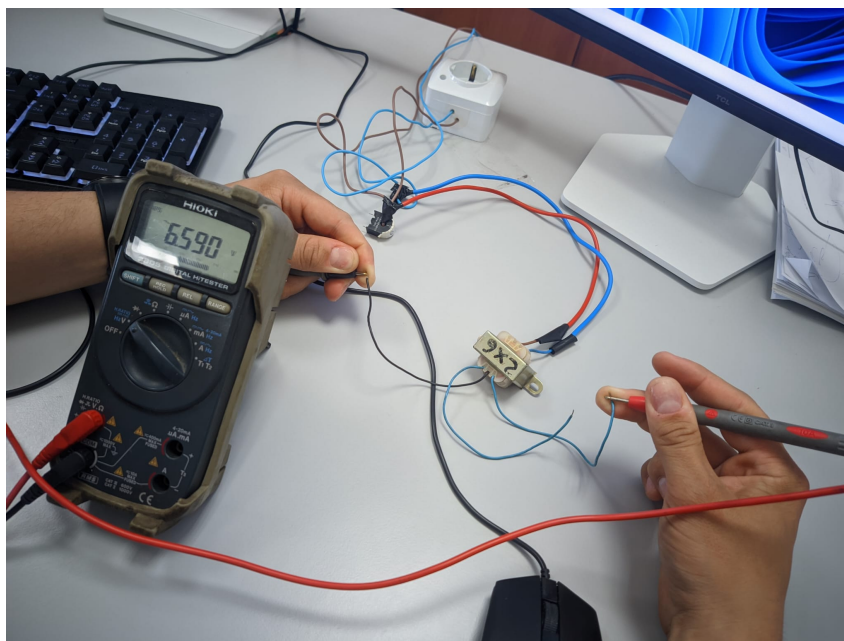
Figura 6. Măsurarea ieșirii transformatorului cu multimetru HIOKI 3805
