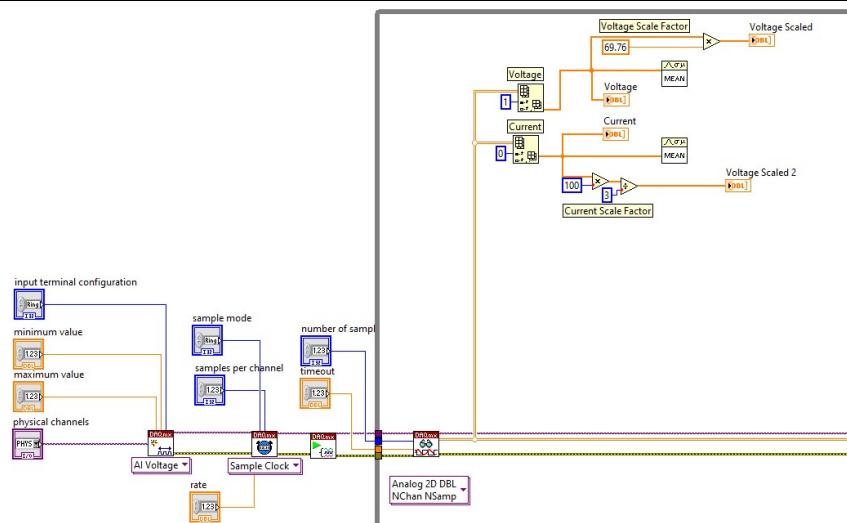
Figura 8. Model VI de testare și vizualizare a semnalului achiziționat
